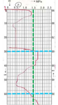
上: 貫入式土壌硬度計による耕盤層の確認 右: 土壌硬度結果
