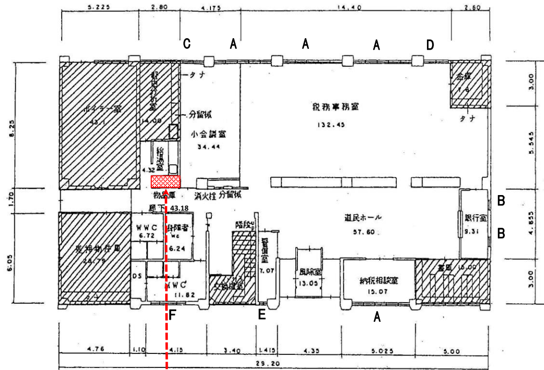
1階平面図
